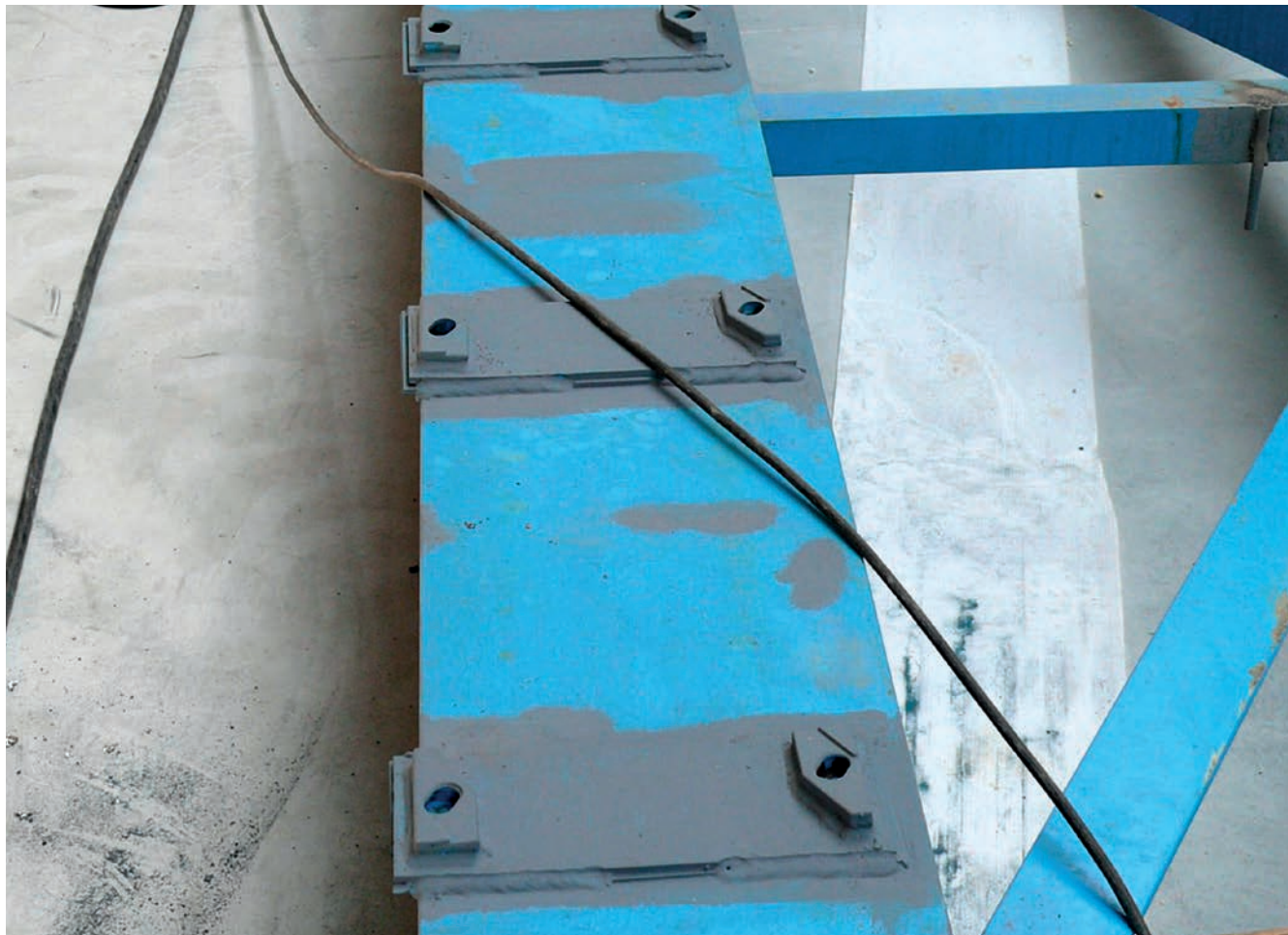
Obr. 5 – Excentrické uložení kolejnice a „vertikální rektifikace“
